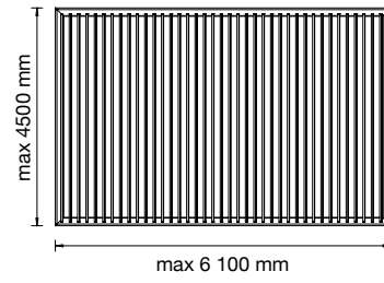
SIMPLE BAIE
