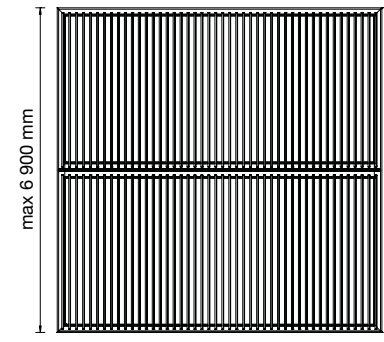
DOUBLE BAIE
