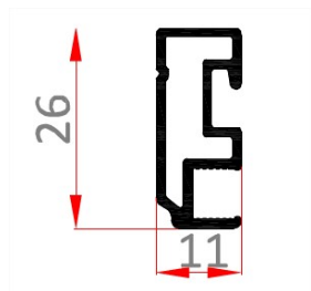
Profil
